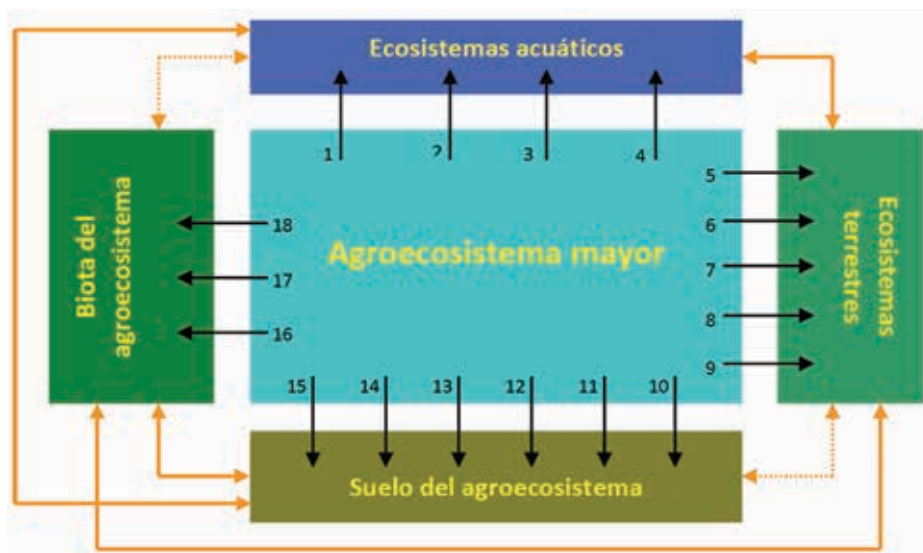
Figura 7. Modelo de impactos ecosistémicos de las prácticas agropecuarias sobre la biodiversidad. Fuente: Silva y Valenzuela (2003).
